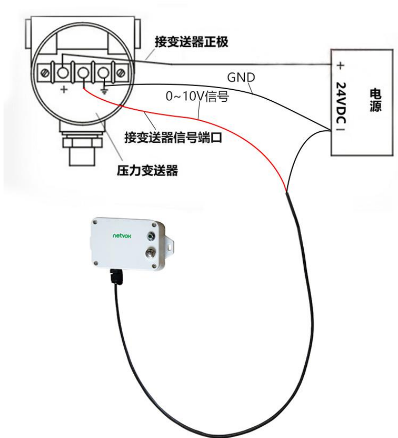
图四 外接 sensor 3 线制接线说明示例图（供接线参考）
